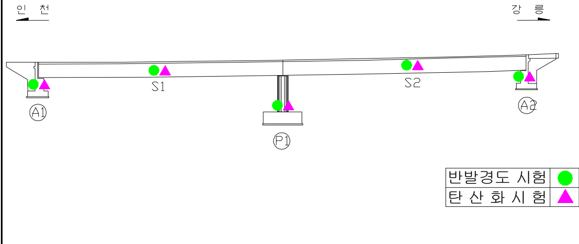
<그림 4.2.1> 재료시험 위치도
